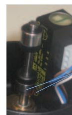
Detektionsscheibe und Schaltnocken für offenes Ventil
