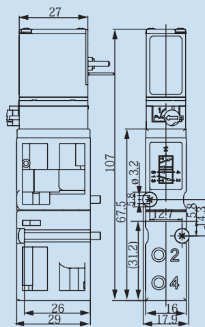
图 2 6527型 两位五通, 回路功能 H
