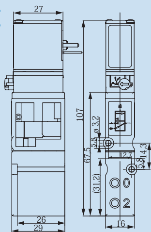
图 1 6526型 两位三通, 回路功能 C
